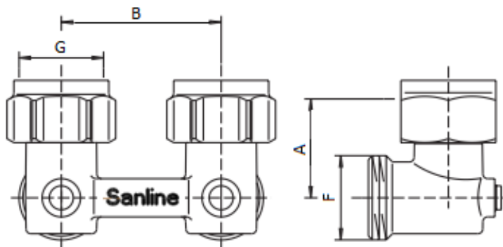
Рис.2 Узел нижнего подключения Н-образный, евроконус G3/4-G3/4, угловой (39103)
