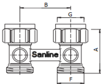
Рис.1 Узел нижнего подключения Н-образный, евроконус G3/4-G3/4, прямой (39101) Узел нижнего подключения Н-образный, евроконус G3/4-G3/4, прямой с байпасом (39102)
