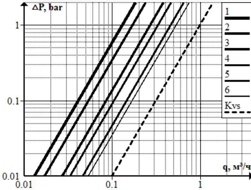
Рисунок 2 – Гидравлические характеристики углового (RA2-15A) клапана
