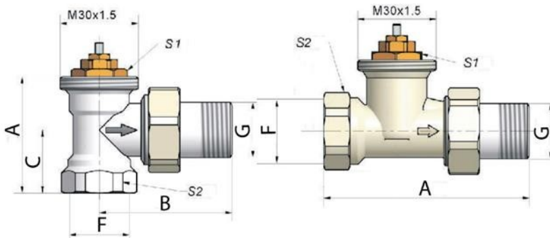
Рисунок 3 – Размеры клапанов
