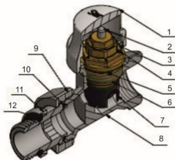
Рисунок 4 – Устройство клапана
