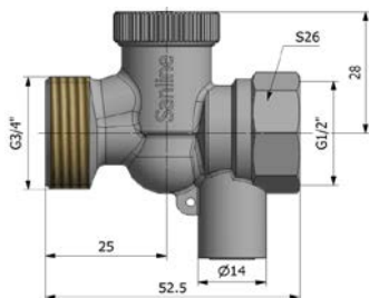
Рисунок 4 – Размеры клапана MRV-15 MRV-20
