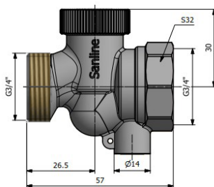
Рисунок 5 – Размеры клапана
