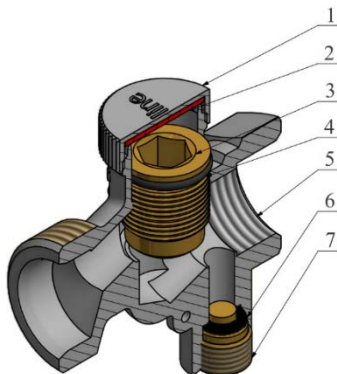
Рисунок 6 – Устройство клапана
