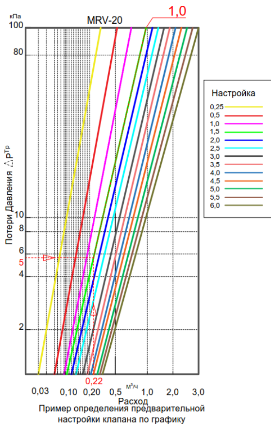
Рисунок 3 – Гидравлические характеристики ручного запорно- регулирующего клапана MRV-20
