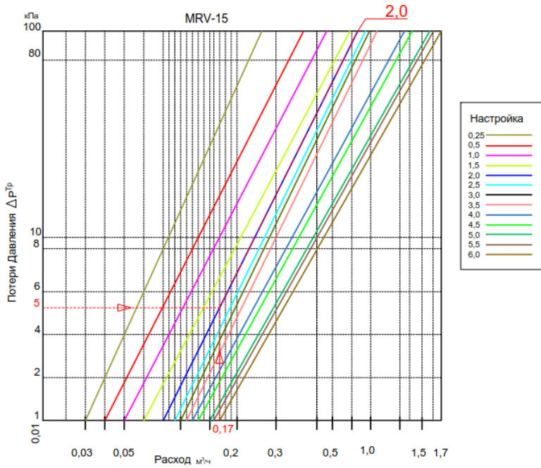
Рисунок 2 – Гидравлические характеристики ручного запорно-регулирующего клапана MRV-15
